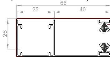
PROWADNICA PODWÓJNA PPD-79 (dotyczy tylko profili PVC-37, PA-39, PA-45)
