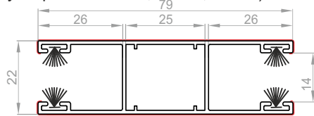
PROWADNICA PODWÓJNA PPD-79 (dotyczy tylko profili PVC-37, PA-39, PA-45)
