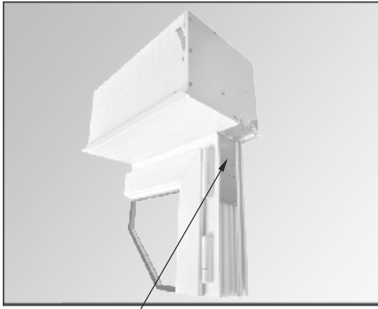
TL1000 Z POSZERZENIEM Minimalna szerokość poszerzenia z napędem to 5,5 cm. Przy zastosowaniu zwijacza podtylnkowego - wyjście taśmy występuje tylko od czoła skrzynki. Poniżej 5,5 cm występuje poszerzenie skrzynki zakończone płytą z pleksiglasu, w którym nie ma możliwości umieszczenia napędu.
